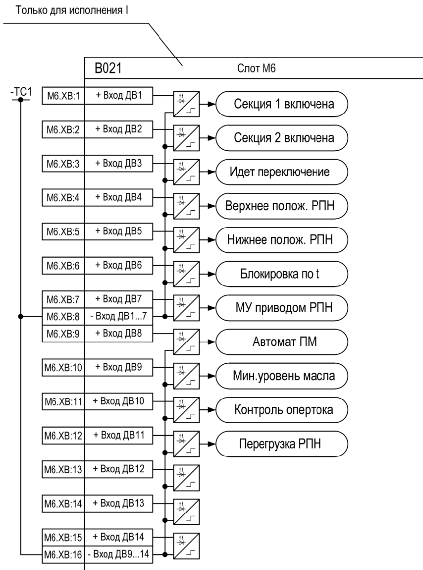
Рисунок Г.2 – Подключение дискретных входов к внутренним сигналам алгоритмов для блоков в слотах М5, М6
