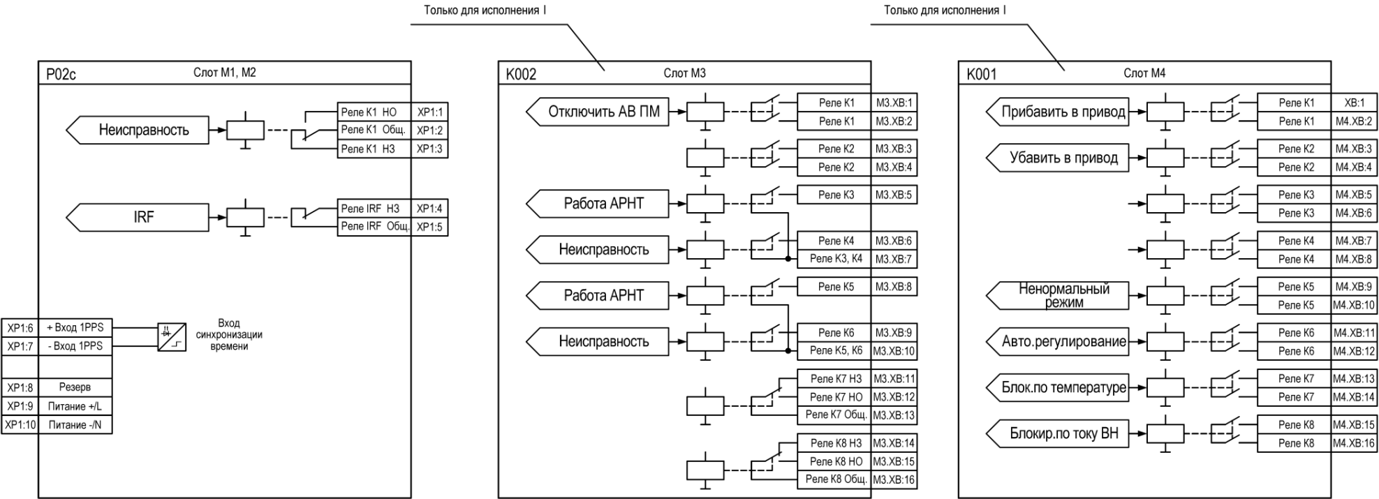
Рисунок Г.1 – Подключение выходных реле к внутренним сигналам алгоритмов для блоков в слотах M1, M3, M4
