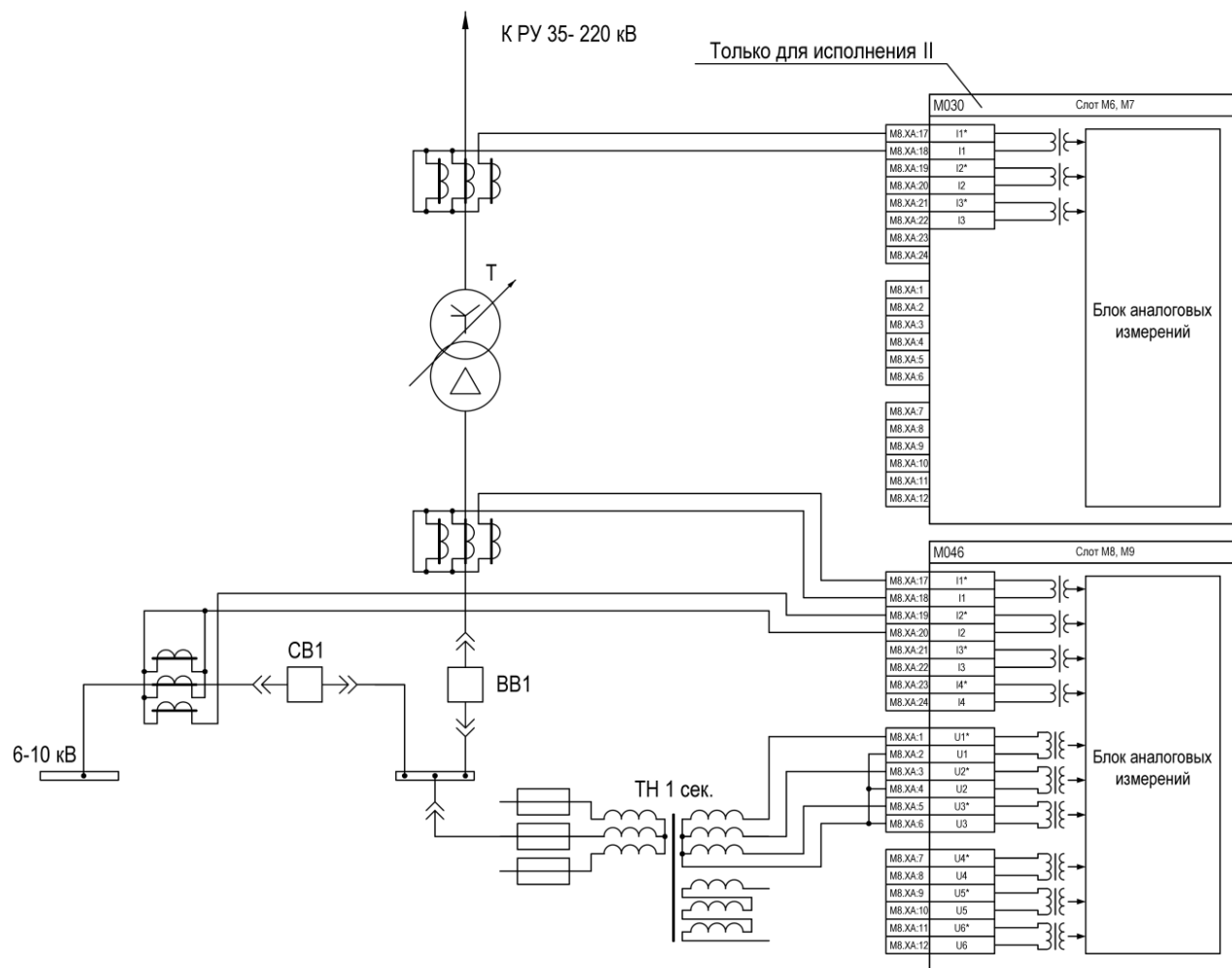
Рисунок В.1 – Подключение цепей ТТ и ТН к измерительному блоку устройству (в случае двухобмоточного трансформатора)
